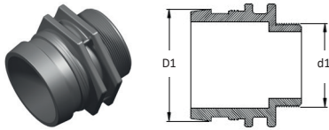
Redüksiyon Nipel (Dişli) / Reduction Nipple (Threaded)
