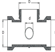
Dişi X Erkek TE / Female X Male TE
